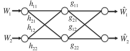
그림 2. 2-셀 2-홉 스몰셀 무선망.
